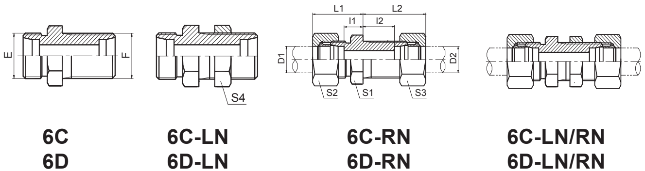
直通过板接头 STRAIGHT BULKHEAD FITTINGS
